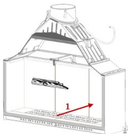
1. Wprowadzić lewą część deflektora do komory spalania
