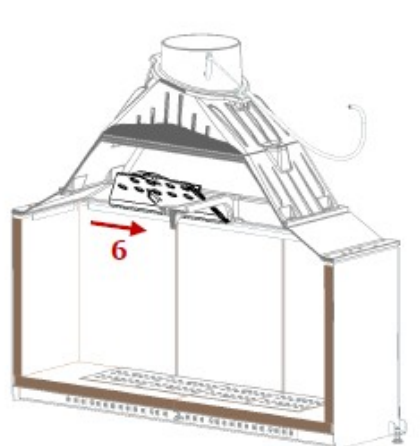
6. Przesunąć deflektor w prawo
