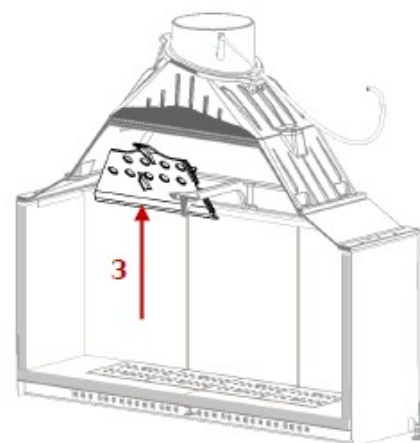
3. Unieść deflektor do czopucha
