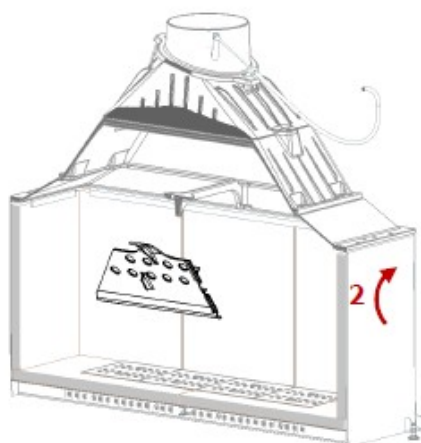
2. Ustawić deflektor pionowo
