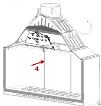
4. Oprzeć deflektor na górnej krawędzi cegieł szamotowych
