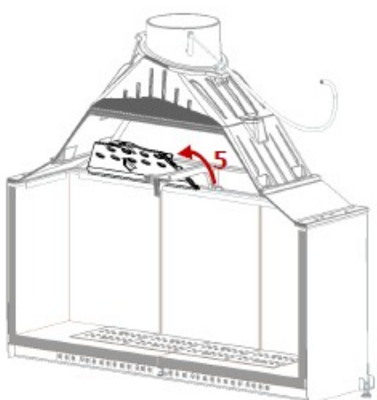
5. Oprzeć przód deflektora o przód czopucha
